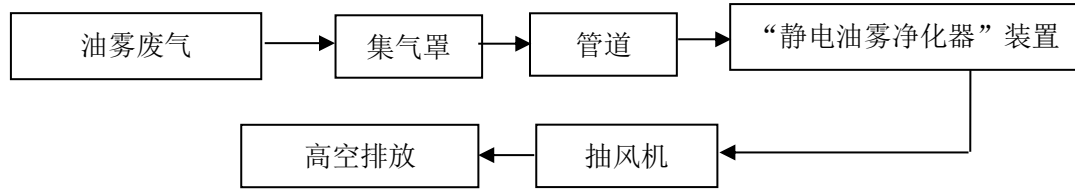
图 4-1 项目废气处理工艺流程图
